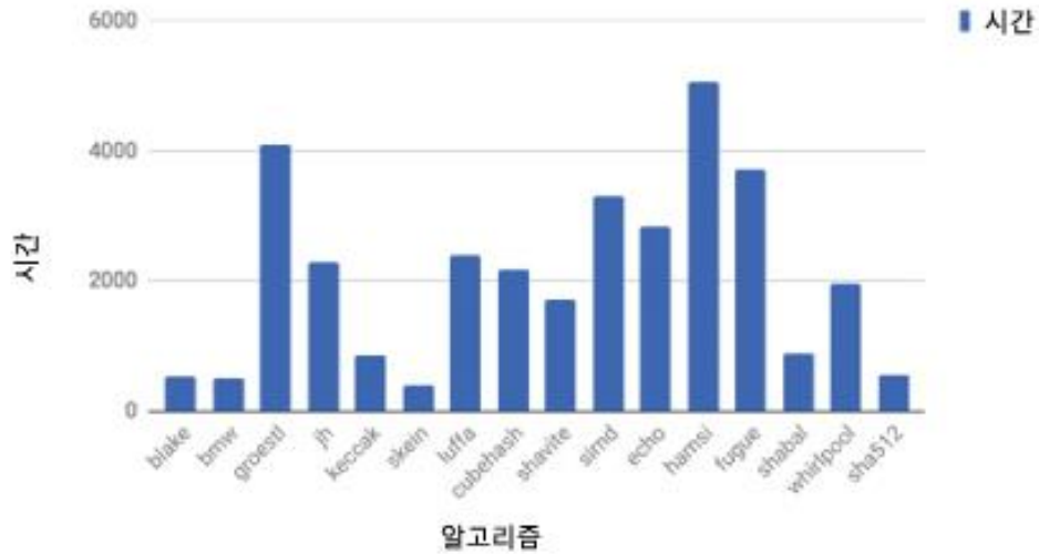
해시 알고리즘당 상대적 출현 시간
